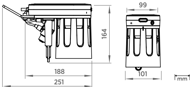
MD30 の寸法
